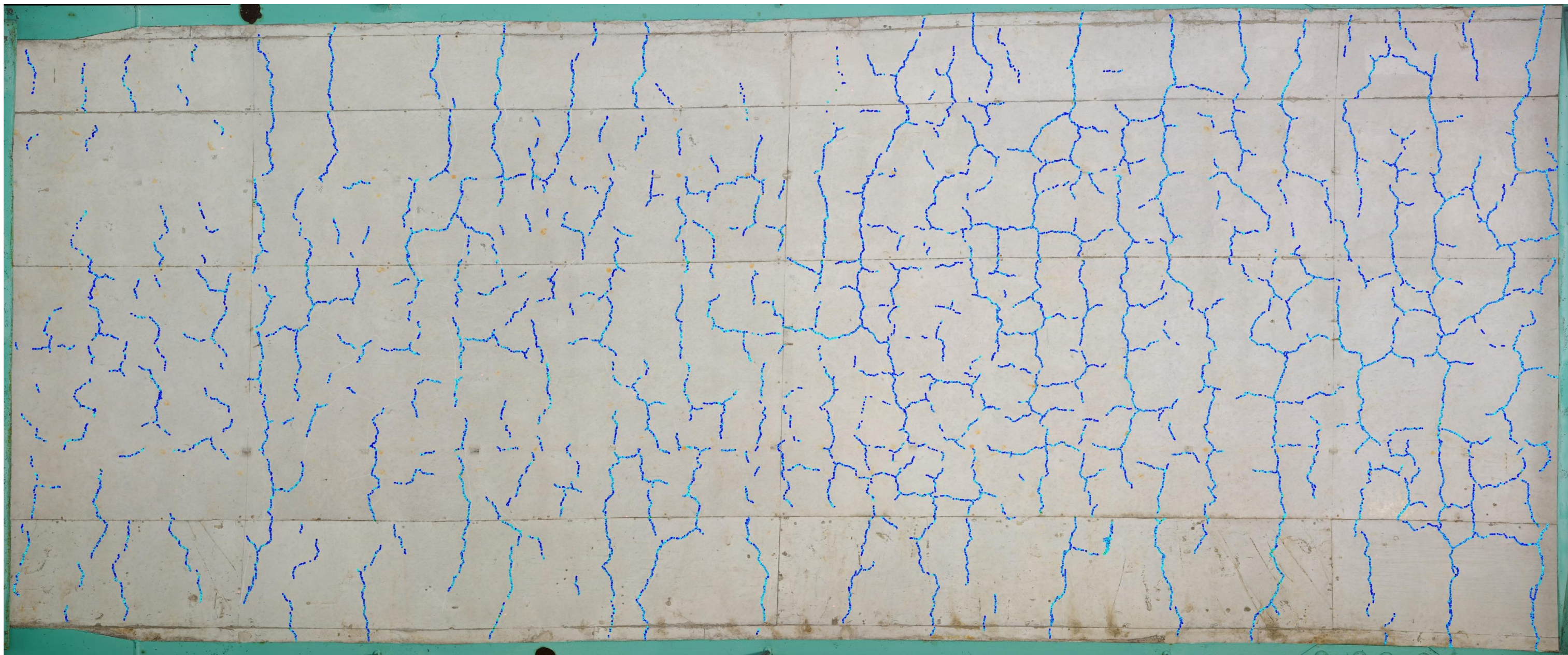
橋梁点検クラック分布図
